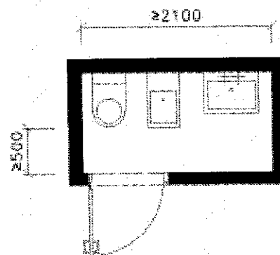
b) Kabina s dveřmi otvírajícími se ven
