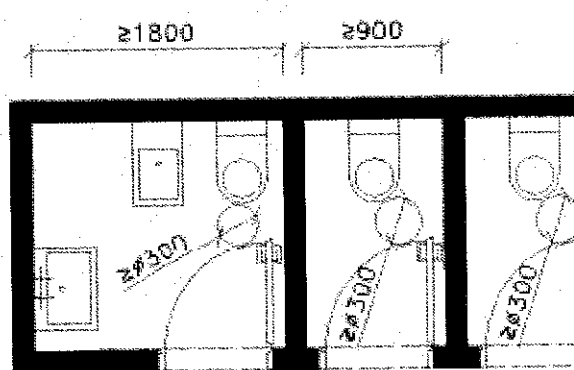
a) Kabina s dveřmi otvírajícími se dovnitř
