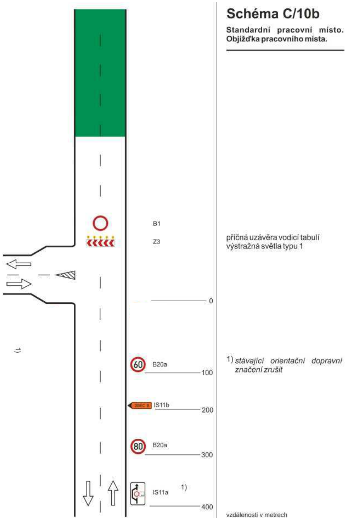
Modifikované schéma C/10 b, snížení rychlosti značením B20a se předpokládá pouze ze směru od Štěchovic, Značení C2b a C2c (které je součástí C/10b dle TP 66) se nenavrhuje
