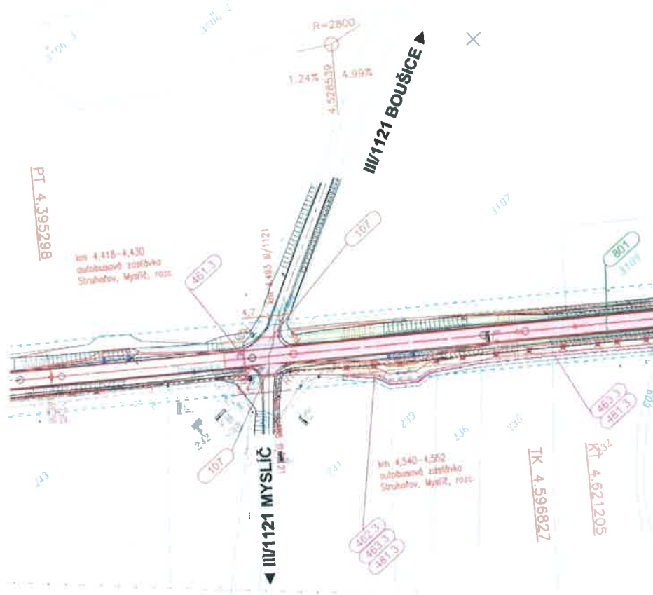
Návrh křižovatky II/112 x III/121
