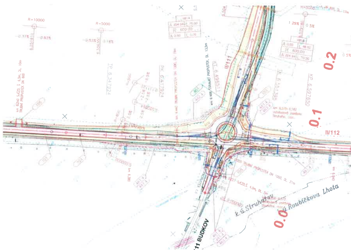
Návrh okružní křižovatky II/112 x II/111
