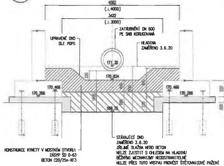
PODÉLNÝ ŘEZ 1:50 V OSE MOSTU
