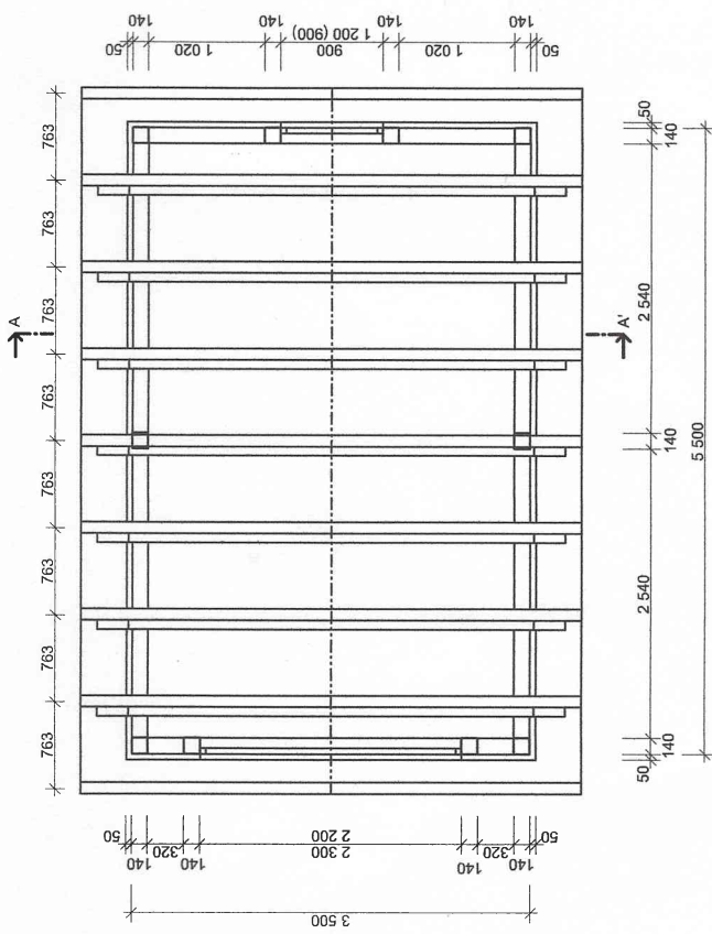
PŮDORYS
