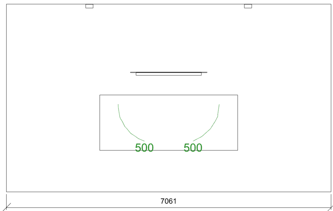
tabule - Normálová osvětlenost 5.36.4 - černé, zelené a bílé tabule - učebna 2 - tabule
