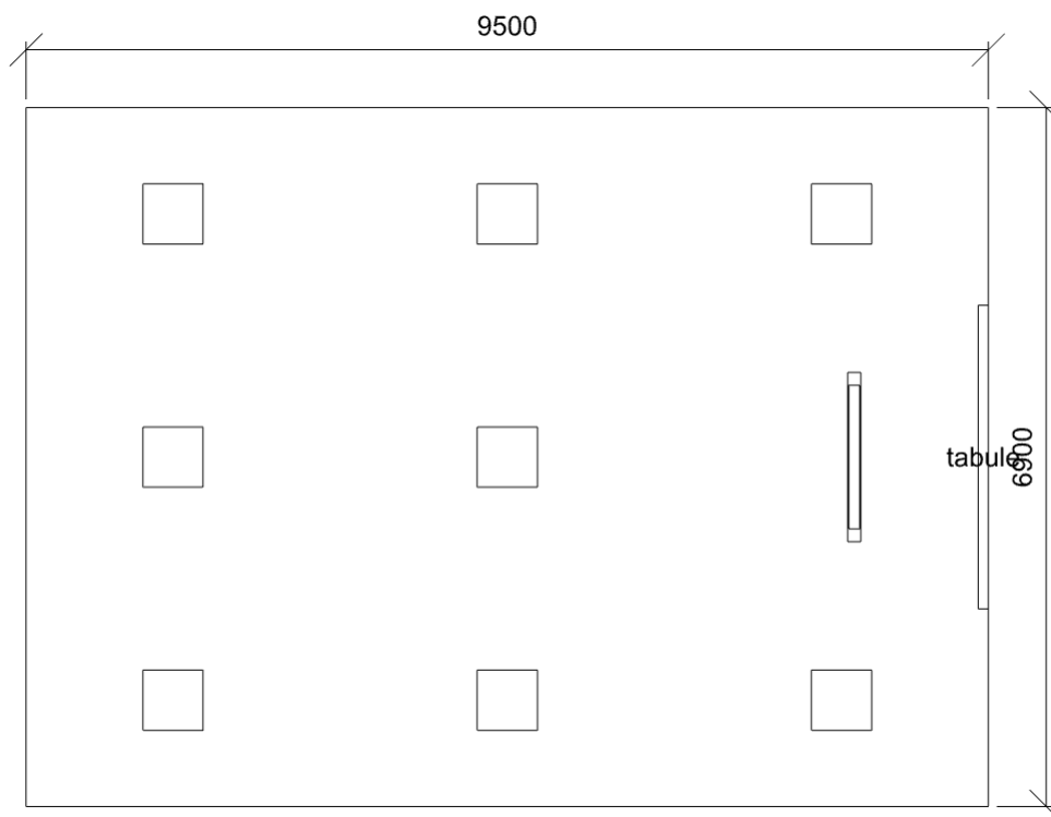
tabule - Normálová osvětlenost 5.36.4 - černé, zelené a bílé tabule - učebna 3 - tabule
