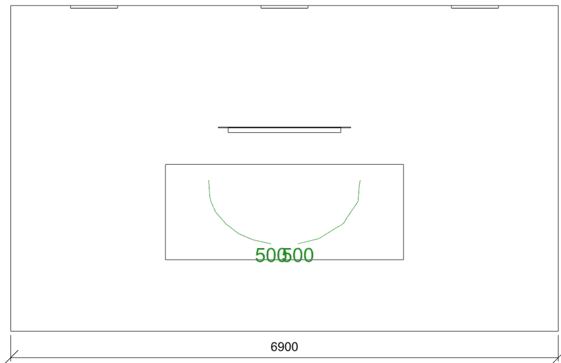
tabule - Normálová osvětlenost 5.36.4 - černé, zelené a bílé tabule - učebna 3 - tabule
