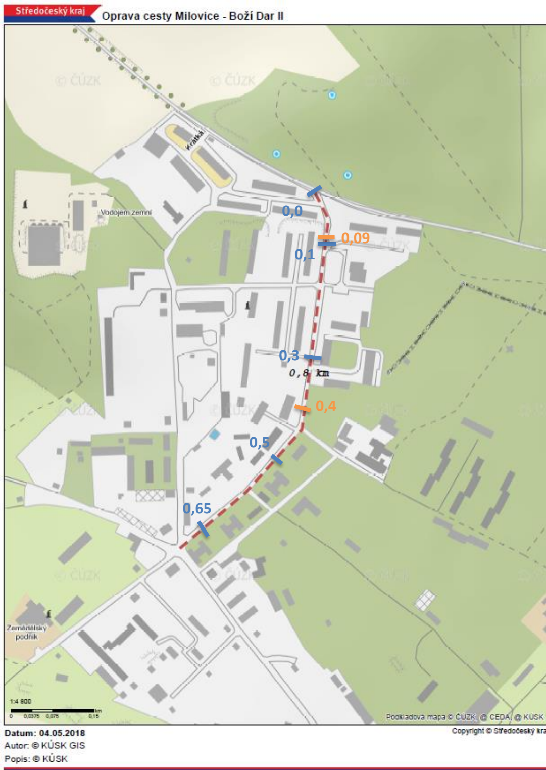
Obr. 1: Obec Milovice – část Boží Dar s vyznačením úseku komunikace, která byla předmětem průzkumu (červenou čárkovanou čarou), umístění vrtů do vozovky (modrou barvou) a kopaných sond (oranžovou barvou)
