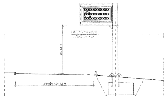
VZOROVÝ PŘÍČNÝ ŘEZ 1:100 (VE SMĚRU STANIČENÍ KOMUNIKACE)
