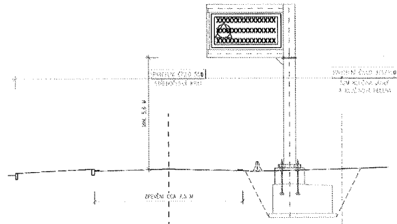
VZOROVÝ PŘÍČNÝ ŘEZ 1:100 (PROTI SMĚRU STANIČENÍ KOMUNIKACE)
