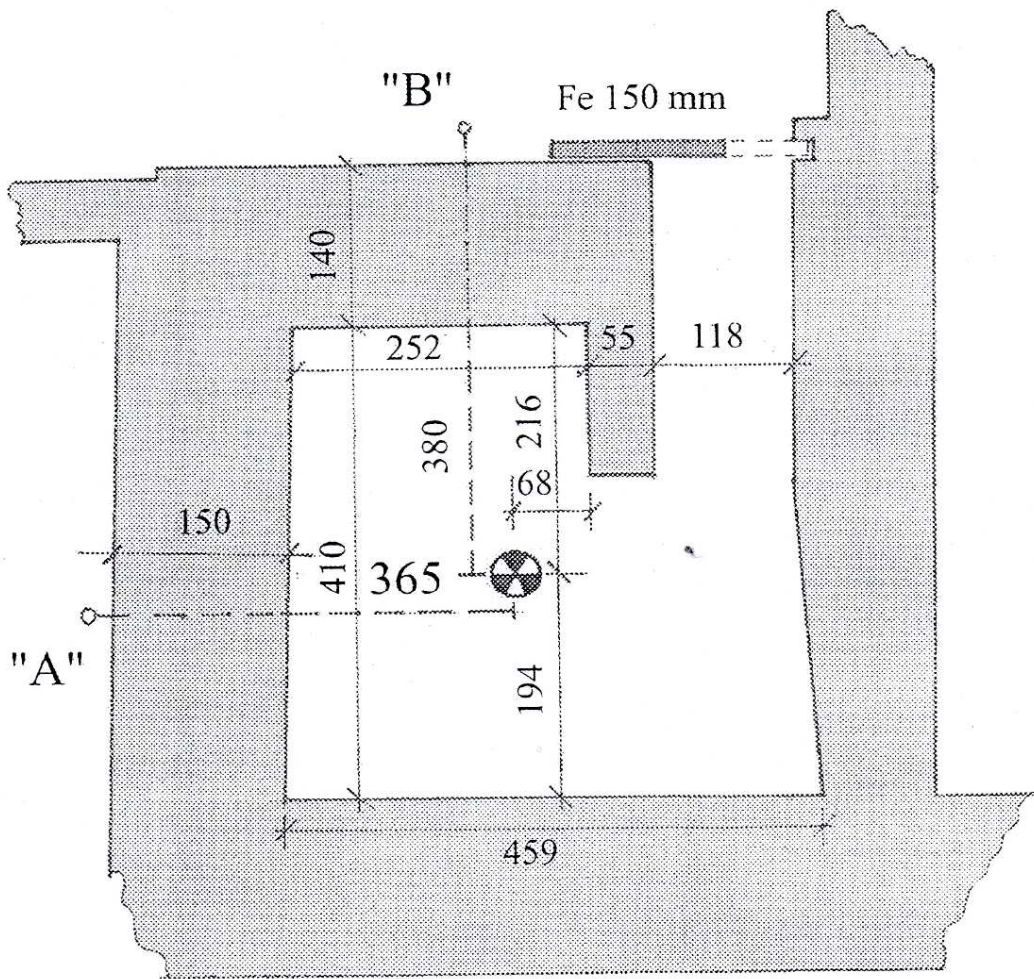
Obr. 1 Půdorys ozařovače Středočeského muzea v Roztokách u Prahy
