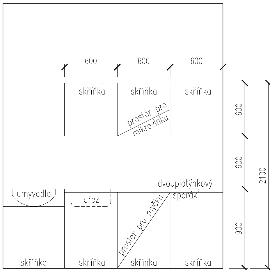
pohled na kuchyňskou linku č.m. 1.04
