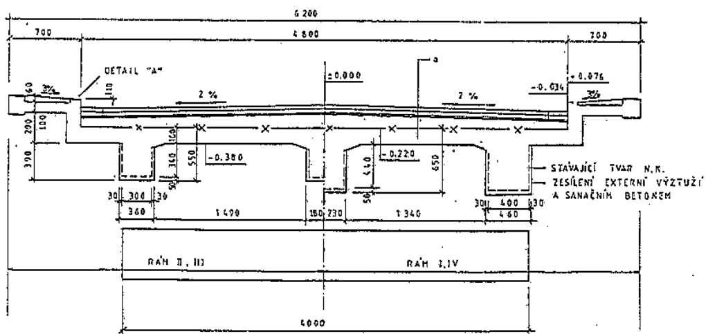
Schematický náčrt mostu, převzatý z ML
