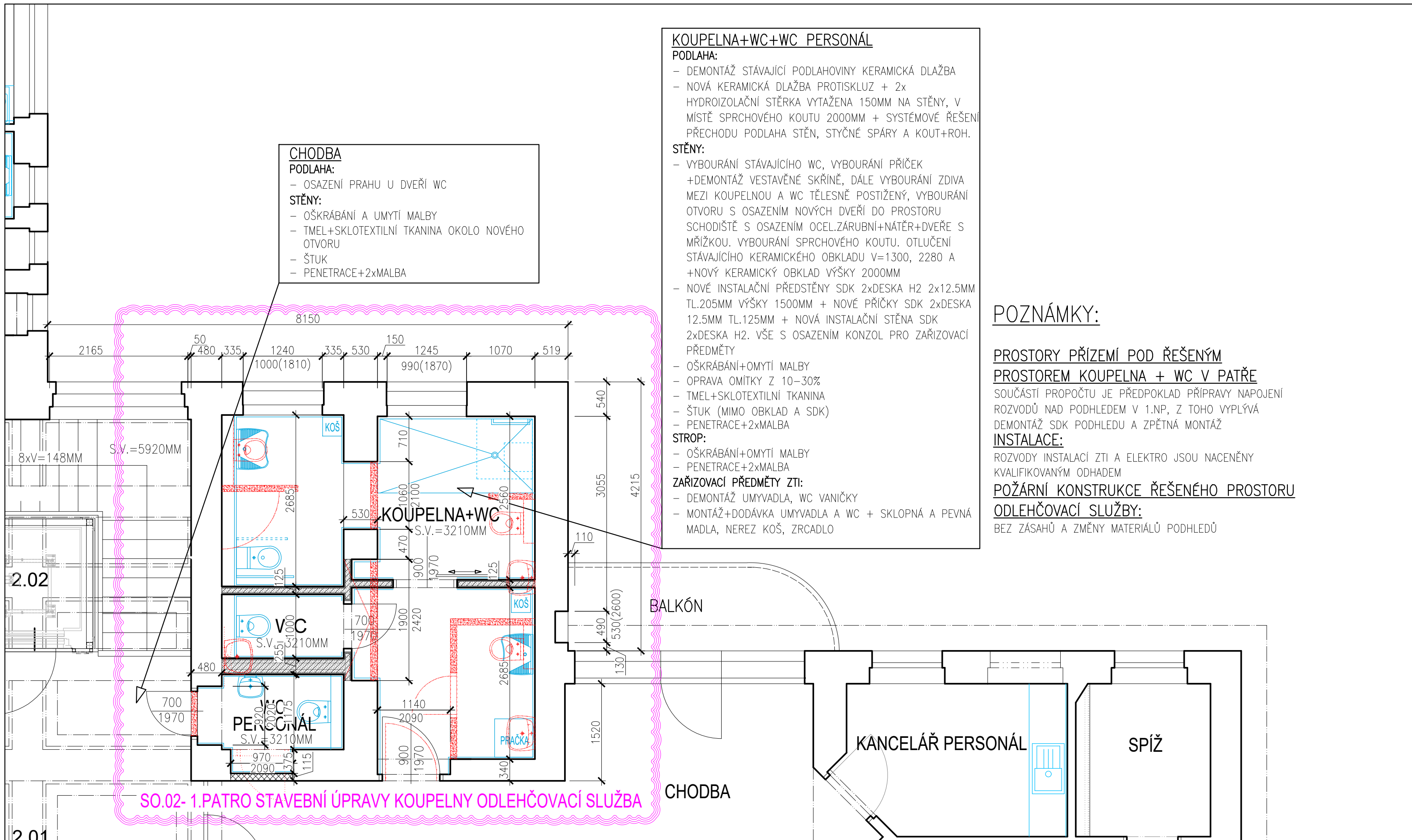
PODKLAD PRO ROZPOČET SO.02 1.PATRO STAVEBNÍ ÚPRAVY KOUPELNY ODLEHČOVACÍ SLUŽBA OBJEKT CENTRA 83, HAVLÍČKOVA 477, MLADÁ BOLESLAV
