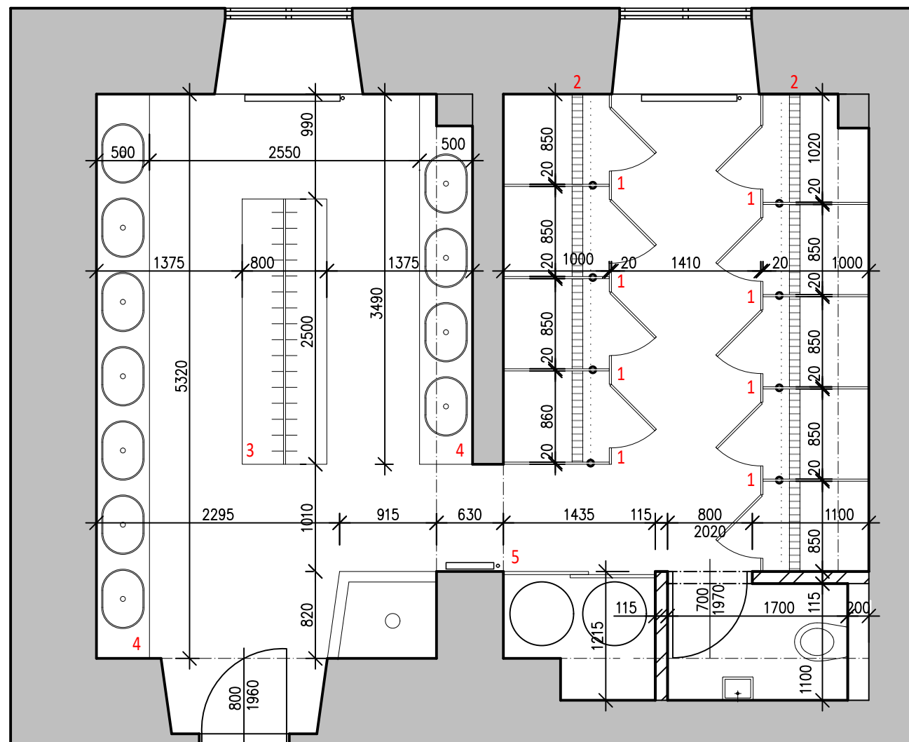
△ PŮDORYS, m 1:50
