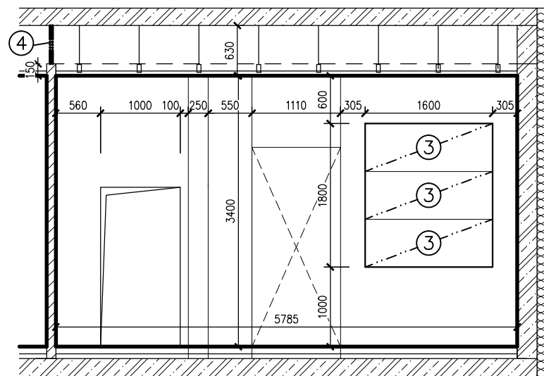
POHLED B-B' (NAPROTI OKNŮM)
