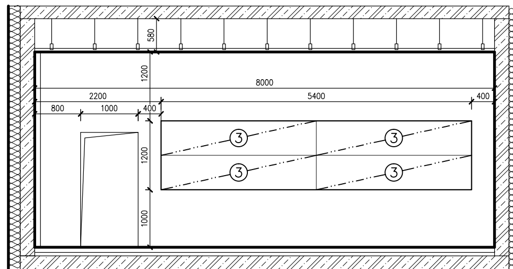
POHLED B-B' (NAPROTI OKNŮM)
