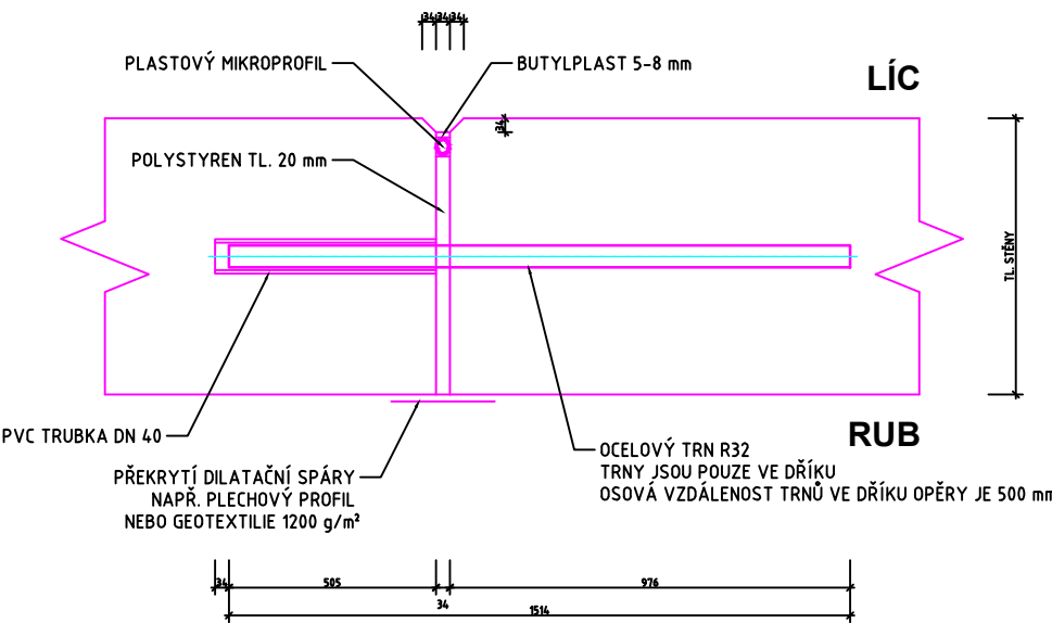
DETAIL DILATAČNÍ SPÁRY
