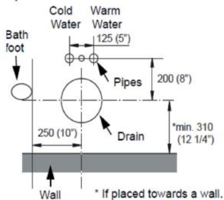
Rozměrový výkres voda-elektro-odpad
