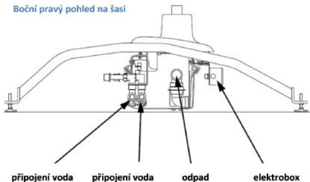
Boční pravý pohled na šasi
