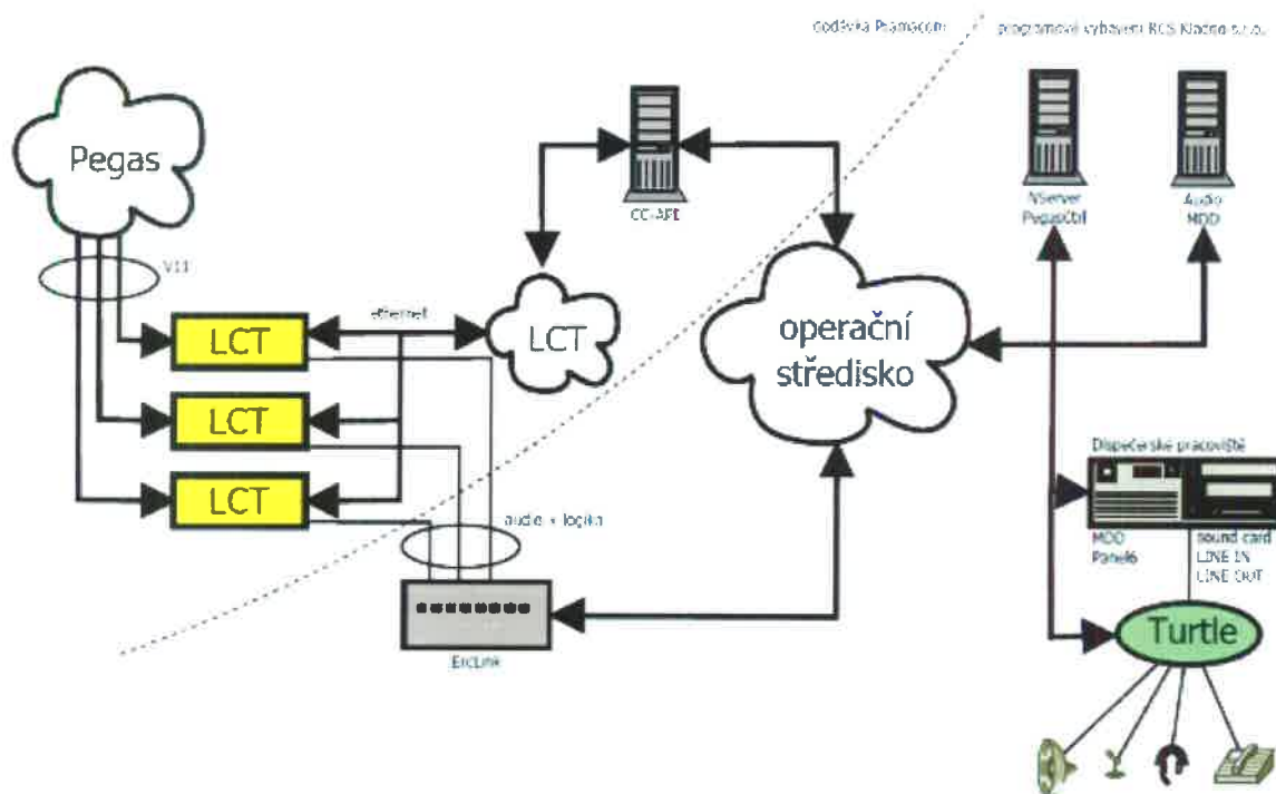
Obrázek 16: Schéma integrace terminálu PEGAS
