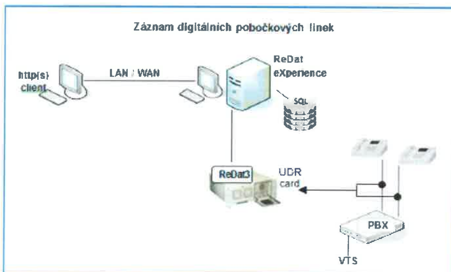
Obrázek 22: Obecný schéma principu záznamu digitálních pobočkových linek.
