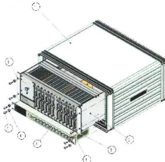
Obrázek 17: LCT RACK
