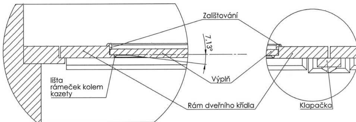
DETAIL B MĚŘÍTKO 1 : 5
